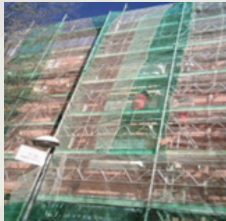
Corregidor Rodrigo Rodríguez, 8 Madrid Aislamiento térmico SATE
