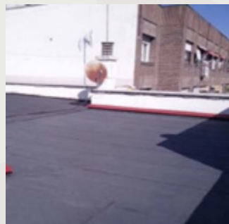
Alustante, 6 Madrid Imprimación asfáltica
