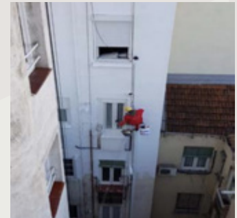
General Pardiñas, 25 Madrid Consolidación de desprendimientos mediante revestimiento petreo
